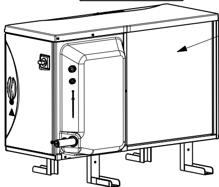
Ech: 1/20 MONTAGE AU SOL FLOOR MOUNTING
